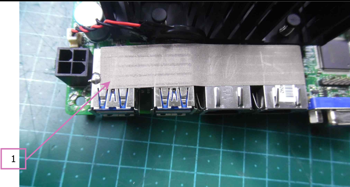
1. 통신포트 접지 보강
