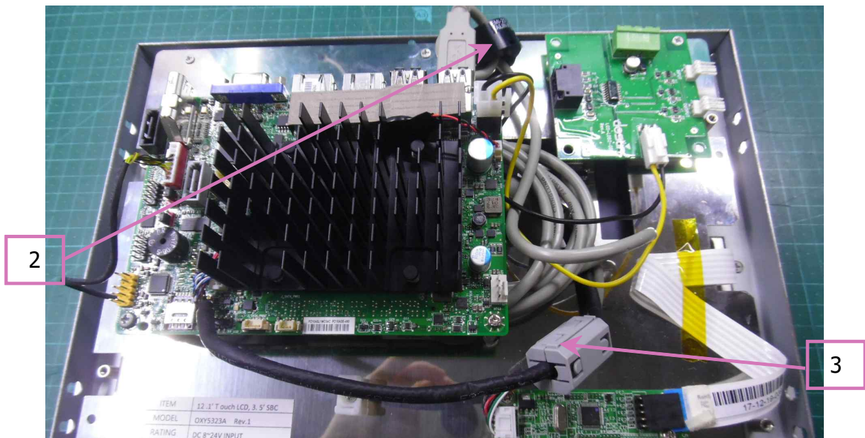
2. 모니터케이블 페라이트 코어 적용 (FEELUX사 BNF-14)
